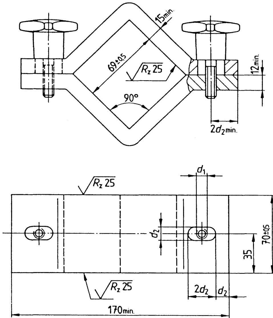
d_2 - średnica przewodnicy
